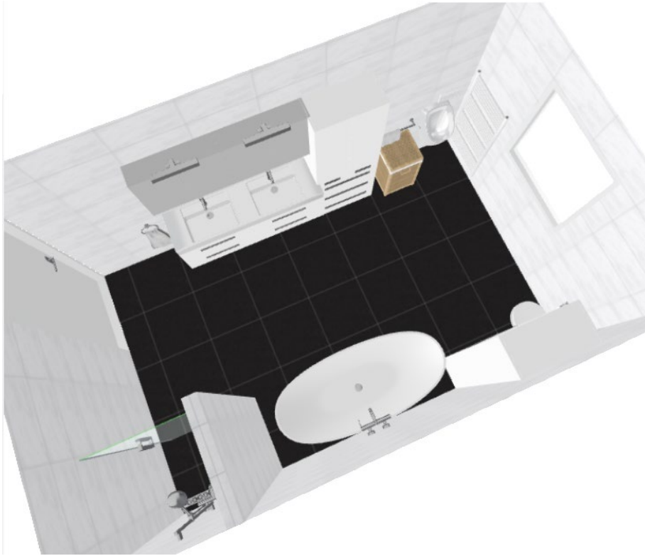
3D-tekening van de badkamer van de familie Batista
